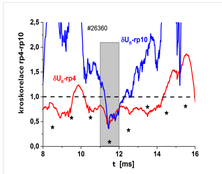
Obrázek 4.22: Časový vývoj relativních fluktuací plovoucího potenciálu U_{fl} měřeného čtvrtým a desátým hrotem. Koeficient vzájemné korelace signálů obou hrotů je označen symbolem \star .
