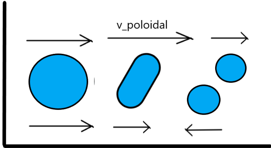
Obrázek 1.3: Vlevo) poloidální rychlost nezávisí na poloměru – nemá stříh. Rozměr turbulentní struktury v okrajovém plazmatu (cca 10 mm) se při poloidální rotaci nemění, plazma spolu s turbulentními strukturami rotuje jako pevné těleso. Uprostřed) poloidální rychlost má stříh, dv_{\text{pol}}/dr je různé od nuly. Turbulentní struktura se v poloidální rovině natočí. Vpravo) velký stříh poloidální rychlosti, v tomto případě v okolí rychlostí stříhové vrstvy. Turbulentní struktura se může rozpadnout na dvě, s menším rozměrem a menší amplitudou.
