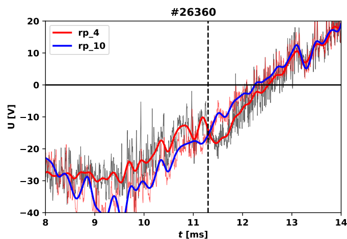
Obrázek 4.20: Časový vývoj plovoucího potenciálu U_{fl} měřeného dvojitou hřebínkovou sondou pro hroty 4 a 10.
