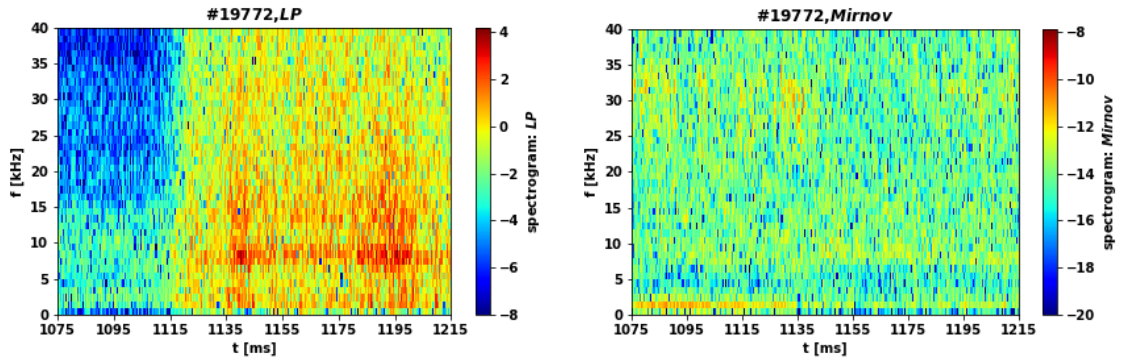
Obrázek 3.25: Vlevo) spektrogram plovoucí Langmuirovy sondy. Vpravo) spektrogram Mirnovovy cívkky.
