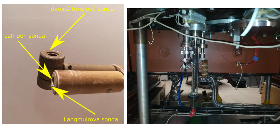
Obrázek 4.1: Schéma tunelové sondy v komoře tokamaku GOLEM nahoře, fotografie kombinované sondové hlavice vlevo, fotografie manipulátoru vloženého do spodního diagnostického portu tokamaku GOLEM vpravo.
