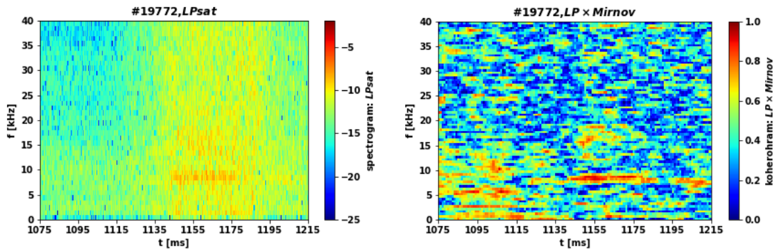
Obrázek 3.26: Vlevo) spektrogram Langmuirovy sondy měřící iontový proud. Vpravo) Spektrum vzájemné koherence Langmuirovy sondy a Mirnovovy cívkky.
