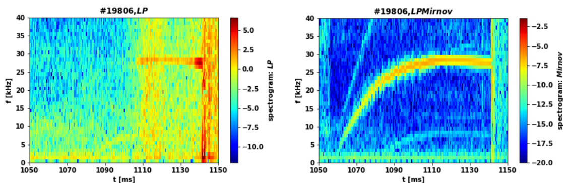
Obrázek 3.50: Vlevo) spektrogram plovoucí Langmuirovy sondy. Vpravo) spektrogram Mirnovovy cívky.
