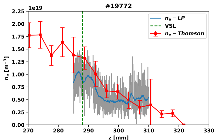
Obrázek 3.15: Radiální profil hustoty plazmatu n_e měřený Thomsonovým rozptylem a Langmuirovou sondou v režimu vysokého záporného napětí, kdy měří iontový proud.
