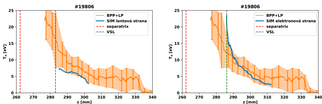
Obrázek 3.43: Vlevo) Iontová strana srovnání elektronové teploty měřené kombinovanou LP a BPP sondou (oranžově) s radiálním profilem elektronové teploty získané srovnáním se simulací (modře). Vpravo) Elektronová strana.
