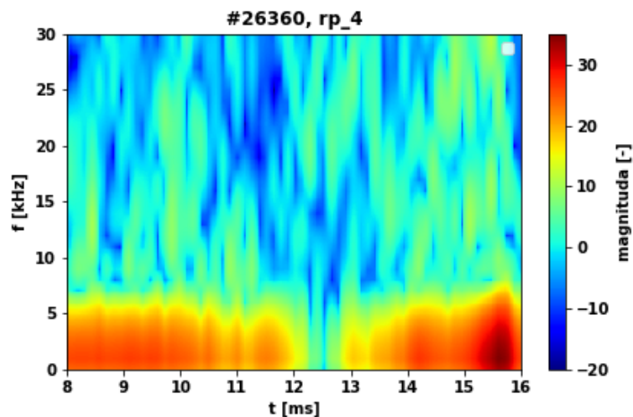
Obrázek 4.23: Spektrogram plovoucího potenciálu U_{fl} měřeného čtvrtým hrotem.
