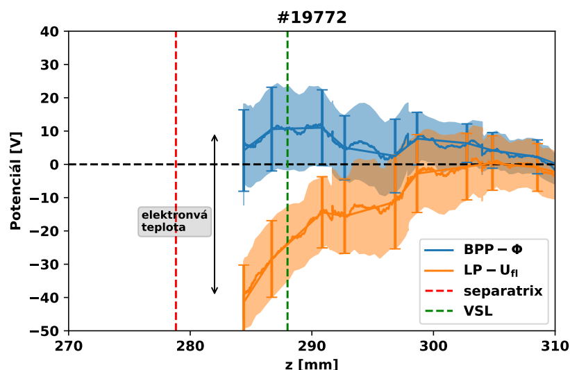
Obrázek 3.8: Radiální profily plovoucího potenciálu U_{fl} měřeného Langmuirovou sondou a potenciálu plazmatu \Phi měřeného ball-pen sondou. Černou šipkou je znázorněn rozdíl potenciálu plazmatu a plovoucího potenciálu, který je úměrný elektronové teplotě. Červenou, čárkovanou čarou je znázorněna poloha separatrix a zelenou, čárkovanou čarou je znázorněna poloha rychlostní stříhové vrstvy (VSL).
