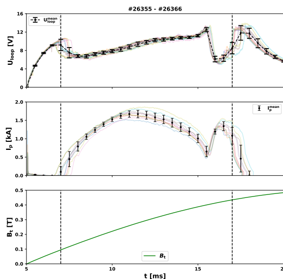
Obrázek 4.17: Základní parametry plazmatu pro výbojovou sérii 26355–26366. Reprodukovatelnost je reprezentována chybovými úsečkami.
