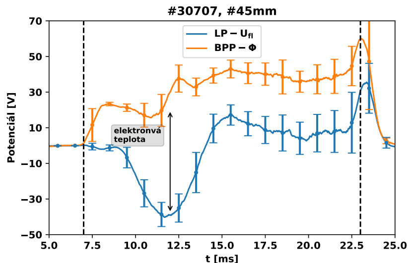
Obrázek 4.13: Časový vývoj potenciálu plazmatu \Phi a plovoucího potenciálu U_f . Rozdíl potenciálů je dle (1.7) úměrný elektronové teplotě.
