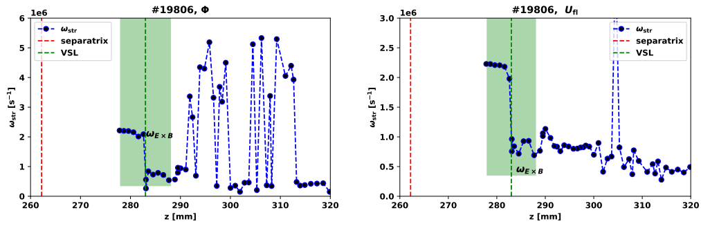
Obrázek 3.46: Profil charakteristické frekvence existence turbulentních struktur \omega_{str} a shearing rate \omega_{E \times B} . Vlevo) potenciál plazmatu, vpravo) plovoucí potenciál.
