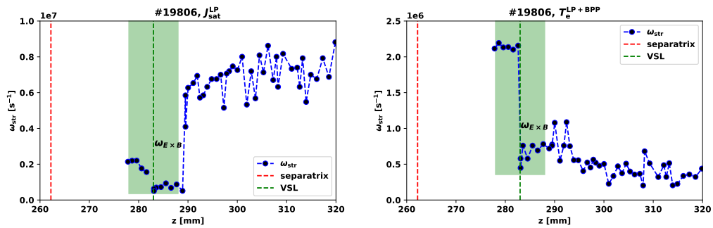
Obrázek 3.47: Profil charakteristické frekvence existence turbulentních struktur \omega_{str} a shearing rate \omega_{E \times B} . Vlevo) hustota iontového proudu, vpravo) elektronová teplota.
