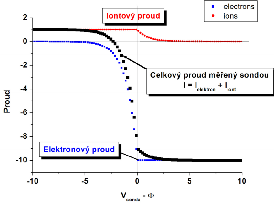
Obrázek 1.1: Ilustrační voltampérová charakteristika. Převzato z [2].
