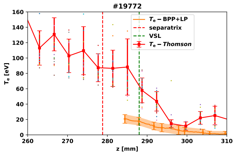
Obrázek 3.10: Srovnání profilů elektronové teploty T_e měřené kombinovanou sondou a Thomsonovým rozptylem. Červenou, čárkovanou čarou je znázorněna poloha separatrix a zelenou, čárkovanou čarou je znázorněna poloha rychlostní stříhové vrstvy (VSL).
