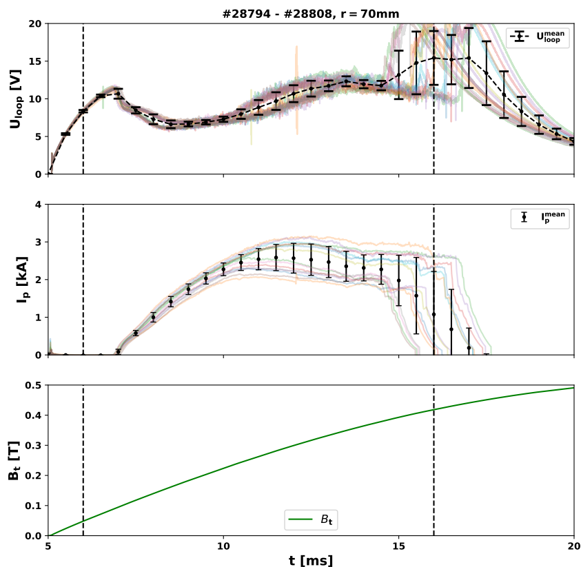
Obrázek 4.3: Základní parametry plazmatu pro výbojovou sérii #28794–#28808 zahrnující proud plazmatem I_p , napětí na závit U_{loop} a toroidální magnetické pole B_t . Reprodukovatelnost výbojové série je reprezentována chybovými úsečkami.
