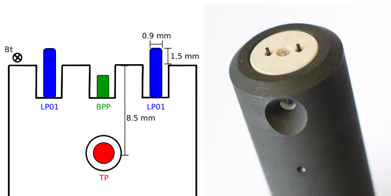
Obrázek 3.1: Schéma a fotografie SEDIBA sondy osazené dvěma Langmuirovými sondami, ball-pen sondou a dvojitou tunelovou sondou. Sonda je umístěna ve vertikálním recipročném manipulátoru.
