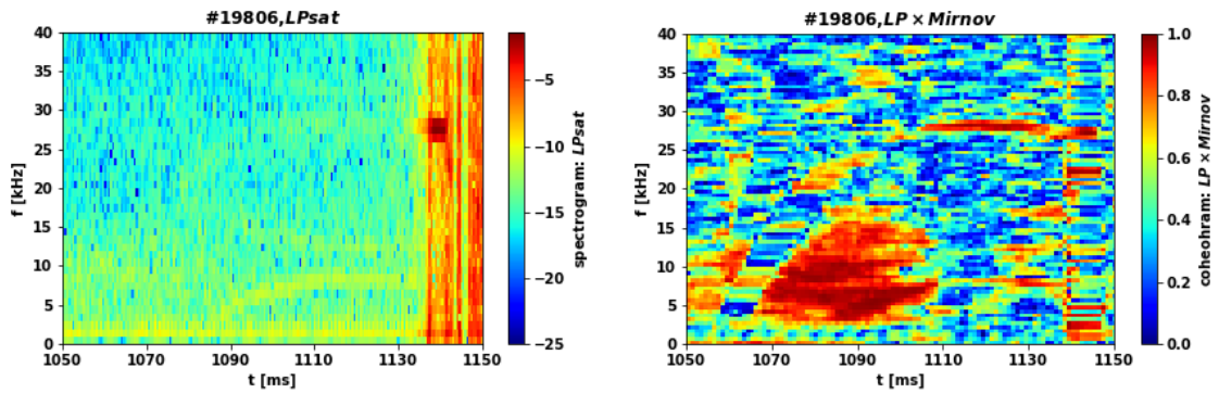
Obrázek 3.51: Vlevo) spektrogram Langmuirovy sondy měřící iontový proud. Vpravo) Spektrum vzájemné koherence Langmuirovy sondy a Mirnovovy cívk.
