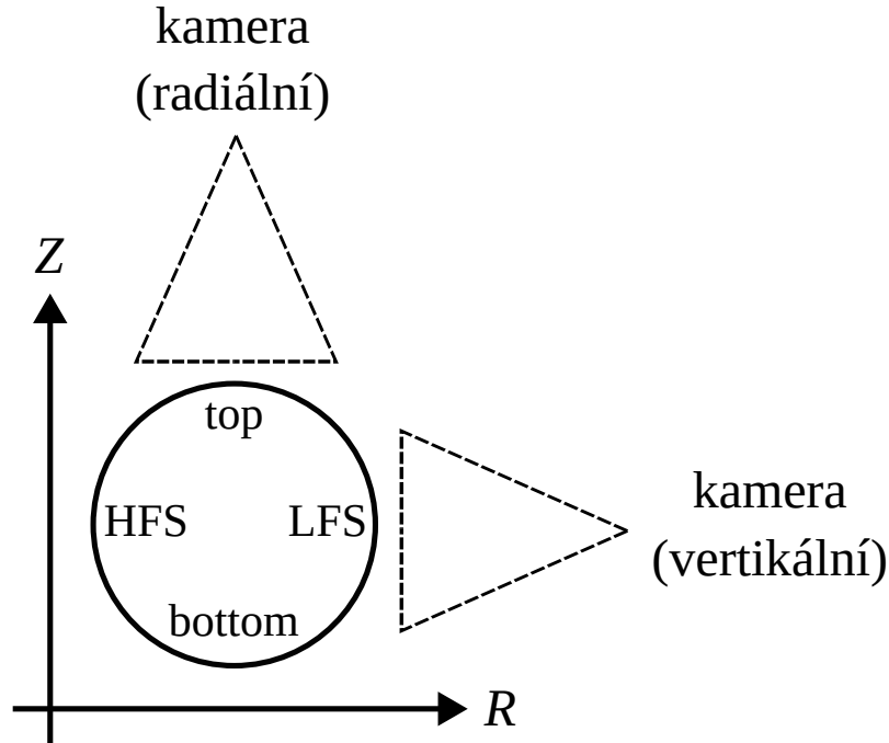
Obrázek 1.6: Schéma umístění dvou vysokorychlostních kamer na tokamaku GOLEM. U obou kamer je uvedeno, jakou snímají polohu plazmatu. Přerušovanou čarou je naznačeno, jakým způsobem kamery snímají obraz.
