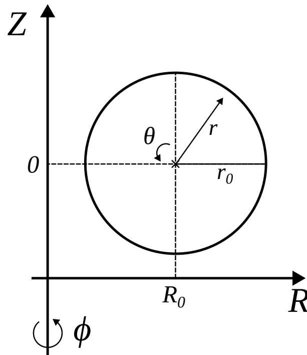
Obrázek 1.2: Schéma poloidálního průřezu s využitím válcového systému souřadnic pro jeho popis (R, \phi, Z) . \phi a \theta značí toroidální a poloidální úhel (resp. směr) a R_0 a r_0 značí hlavní a vedlejší poloměr komory.
