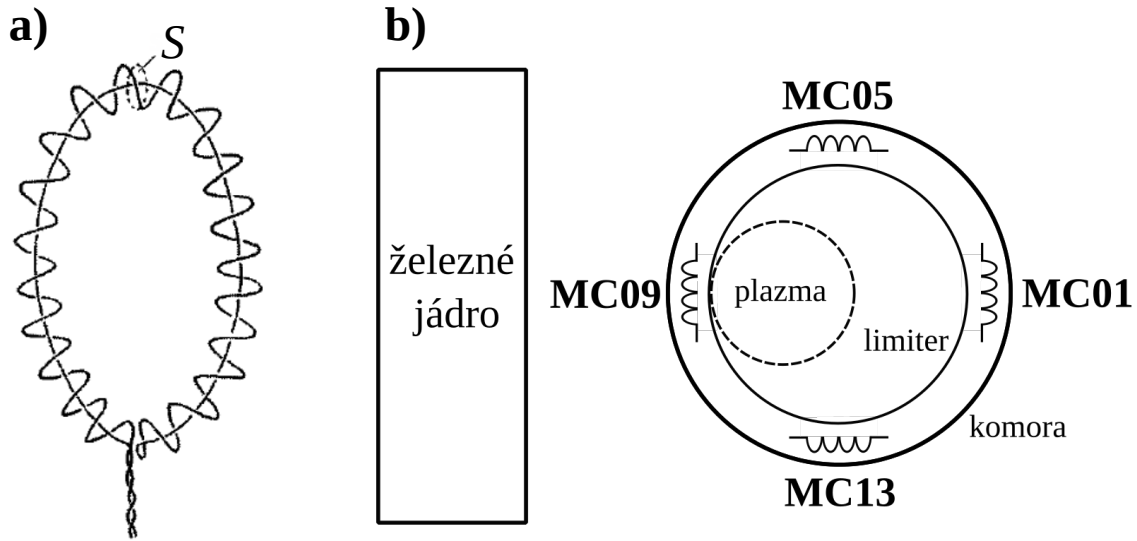
Obrázek 1.5: a) Schéma Rogowské cívy. S značí plochu jednoho závitu cívy, který je orientovaný poloidálně. b) Schéma Mirnovových cívek na poloidálním průřezu. Zdroj obr. a): [19]
