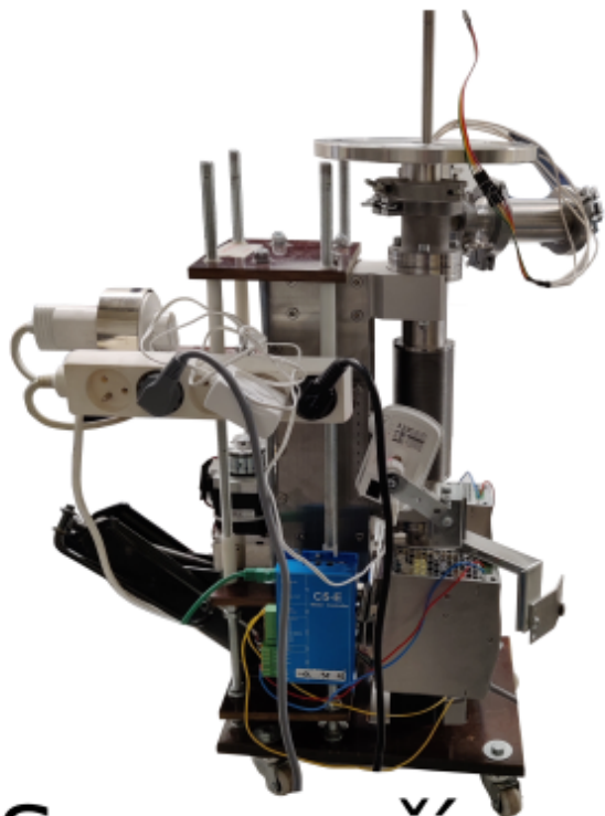
Servem řízený manipulátor
