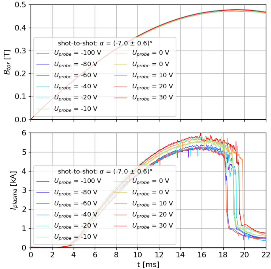
Obr. 3.10: Srovnání reprodukovatelnosti výbojů při měření metodou shot-to-shot. Sledovanými diagnostikami je proud plazmatu I_{plasma} a magnetické toroidální pole B_{tor} .
