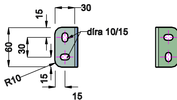
púdorys
