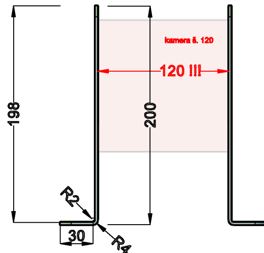
púdorys
