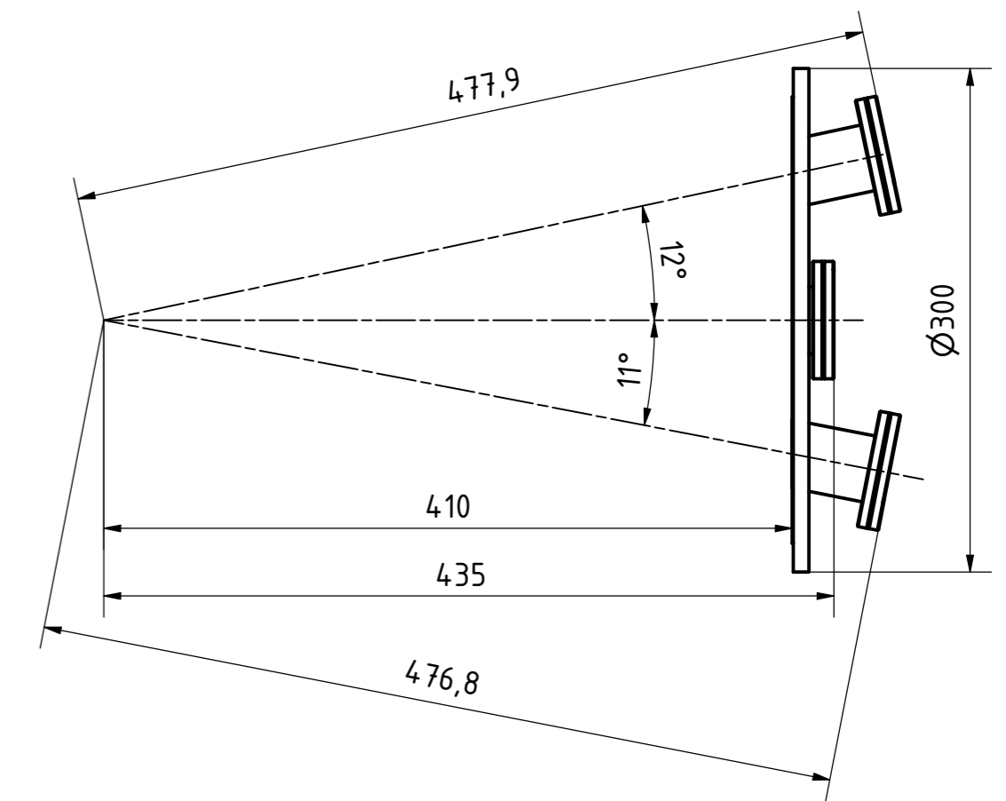
Poloha přírub vůči ohnisku ( 1 : 4 )
