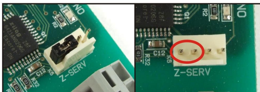
obr. 1 - krátce propojte levé dva piny na konektoru Z-SERV
